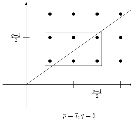
Obr. 4.1: Ilustrácia dôkazu zákona kvadratickej reciprocit, prípad p = 7, q = 5
