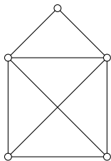
Figure: Príklad grafu s eulerovským ťahom
