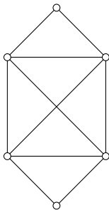
Figure: Príklad grafu s uzavretým eulerovským ťahom
