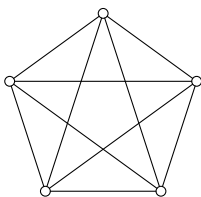
Obr. 9.8: Graf K_5 nie je planárny
