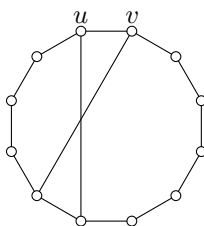
Obr. 9.20: Ilustrácia dôkazu Bondy–Chvátalovej vety
