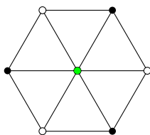
Obr. 9.13: Příklad grafu ofarbeného troma farbami
