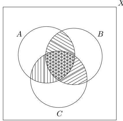
Obr. 5.2: Koľkokrát sme odpočítali jednotlivé prvky
