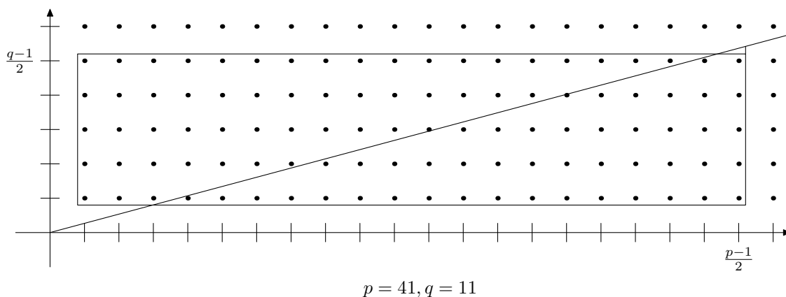
Obr. 4.3: Ilustrácia dôkazu zákona kvadratickej reciprocity, prípad p = 41, q = 11
