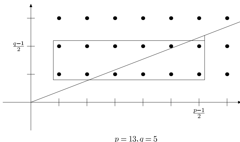
Obr. 4.2: Ilustrácia dôkazu zákona kvadratickej reciprocity, prípad p = 13, q = 5
