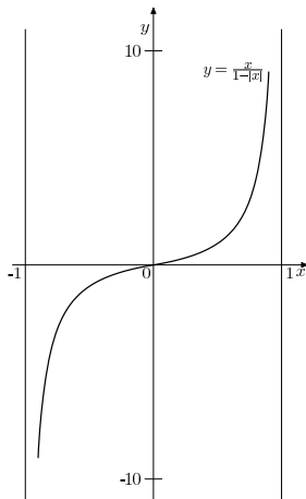
Figure: Bijekcia medzi (-1, 1) a \mathbb{R}
