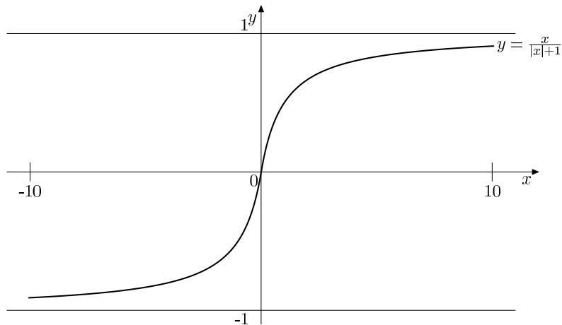
Figure: Bijekcia medzi \mathbb{R} a (-1, 1)
